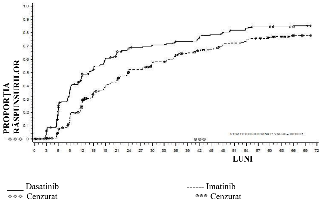
Figura 1: Estimare Kaplan-Meier a timpului până la răspunsul molecular major (RMM)
